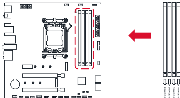
内存安装建议
